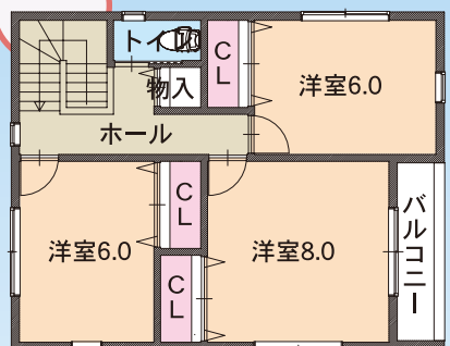
2階平面図
